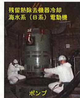
残留熱除去機器冷却海水系 (B系) 電動機 据付作業
