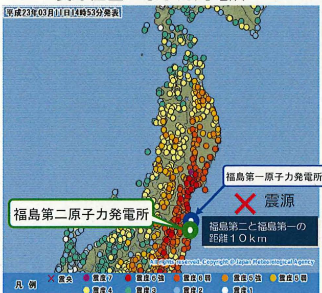
震源位置と原子力発電所
